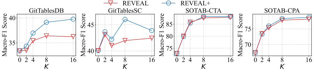
Fig. 8. Vary K .
