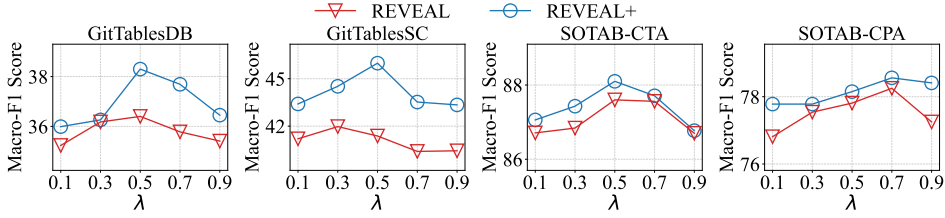
Fig. 9. Vary \lambda .
